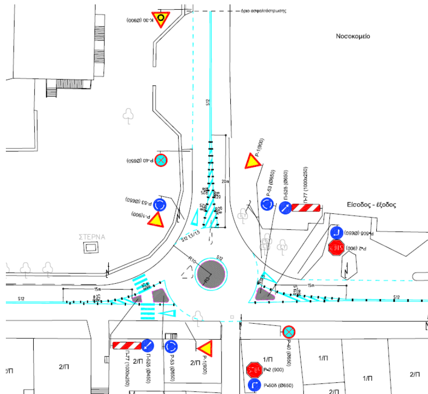
Κυκλικός Κόμβος Κ2 (Απόσπασμα από την εγκεκριμένη μελέτη)
